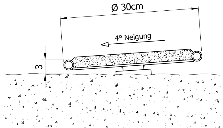
Aufstellung auf losem Untergrund: (wie z.B. Sand, Rindenmulch)
