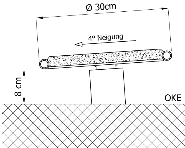
Aufstellung auf festem Untergrund: lichter Mindestabstand: mind. 8cm (wie z.B. Oberboden, Fallschutzplatten u.s.w)
