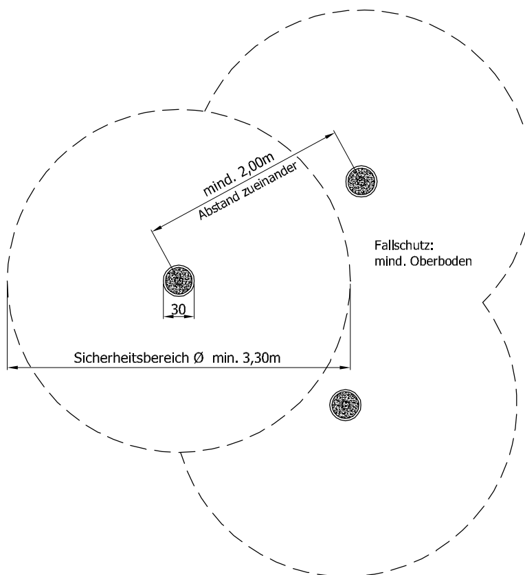
Draufsicht M1:50 -Beispiel Anordnung zueinander-
